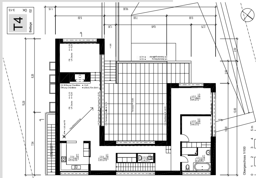
Beilage 02 Obergeschoss 1:100
